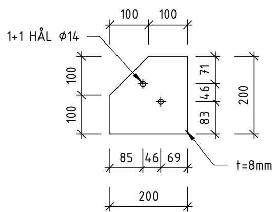
PL01 1 : 10
