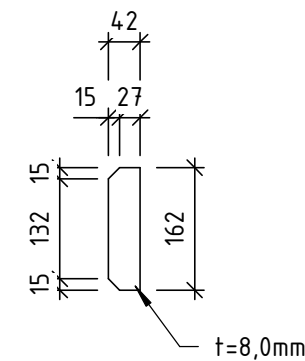
PL06 1 : 10
