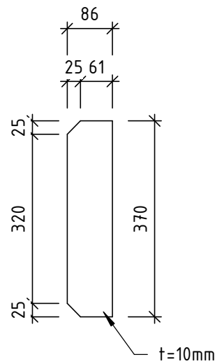
PL04 1 : 10
