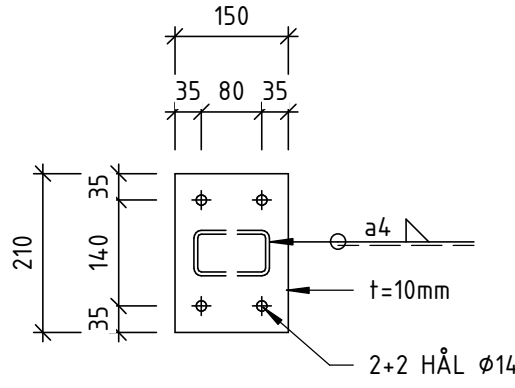
FP03 - PLAN 1 : 10
