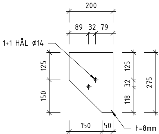
PL02 1 : 10
