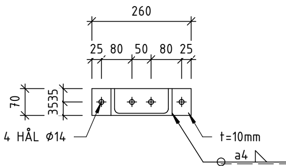
PL05 - PLAN 1 : 10
