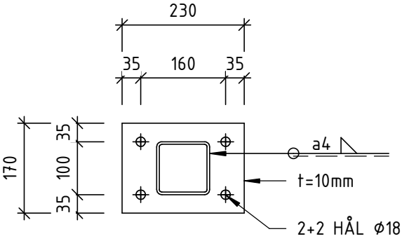
TP01 - PLAN 1 : 10
