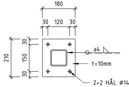
TP04 - PLAN 1 : 10
